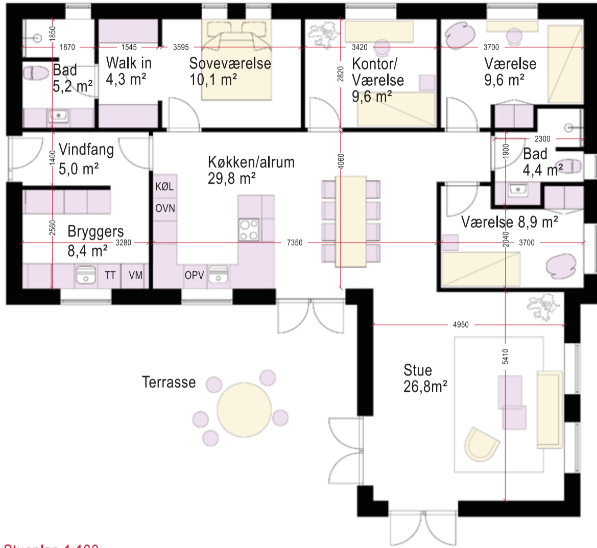
Stueplan 1:100
