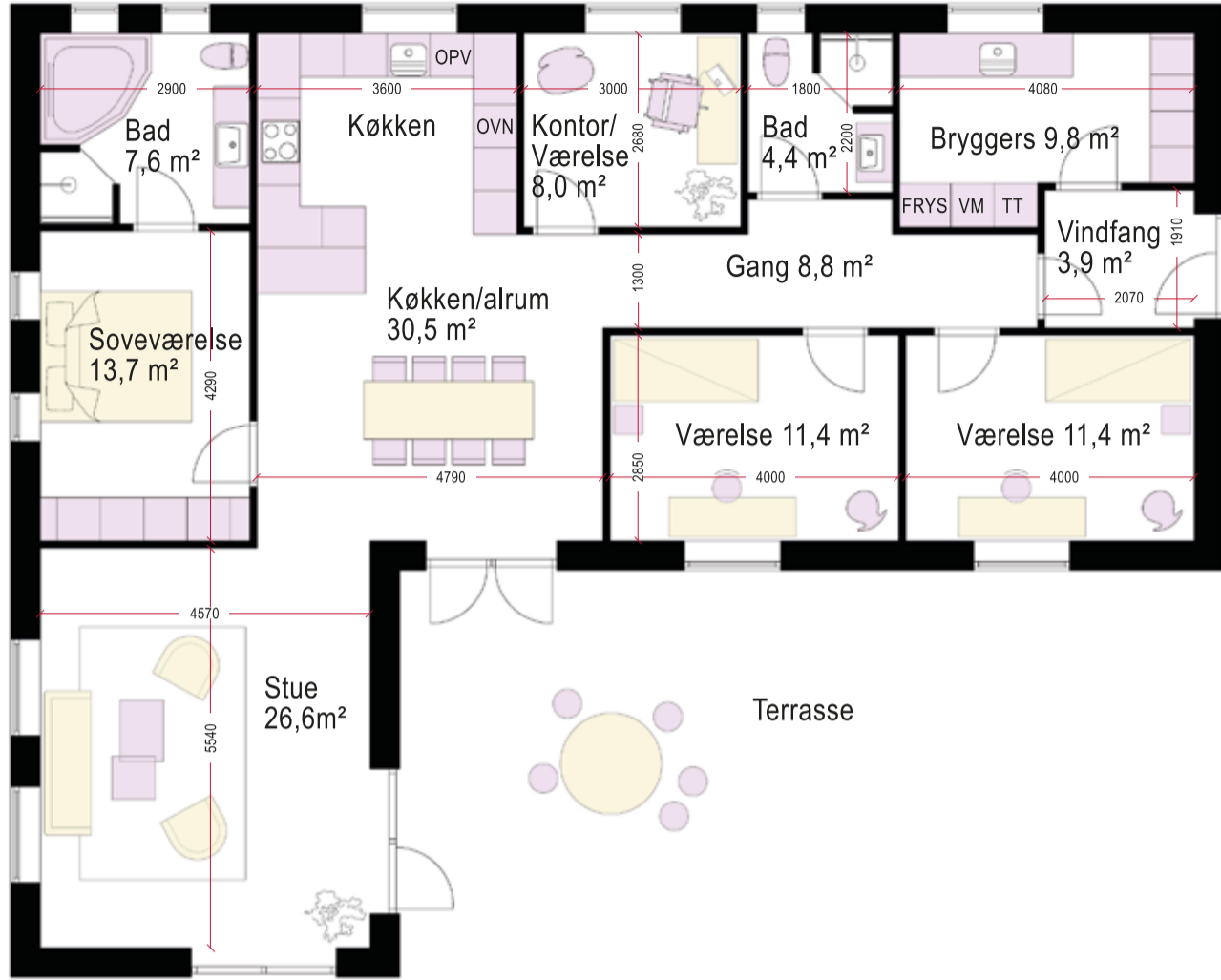
Stueplan 1:100
